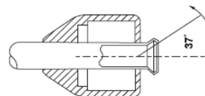
113° - 117° DIN CONVEX TUBE OP.1 OP.2 DIE
