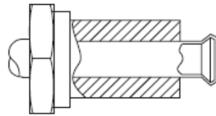
SAE CONVEX TUBE OP.1 DIE
