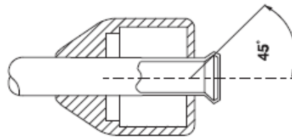
SAE DOUBLE TUBE OP.1 OP.2 DIE
